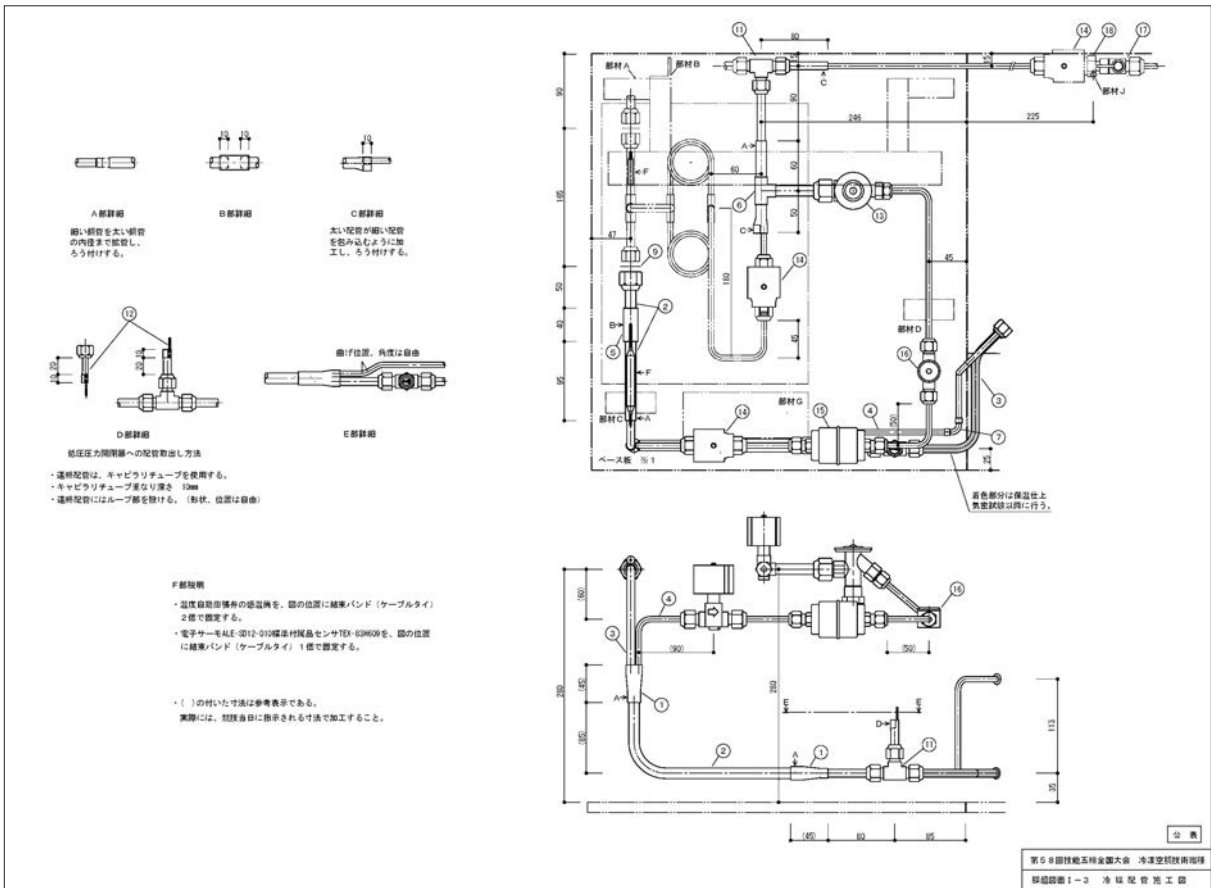
第58回大会 公表課題 冷媒配管施工書
