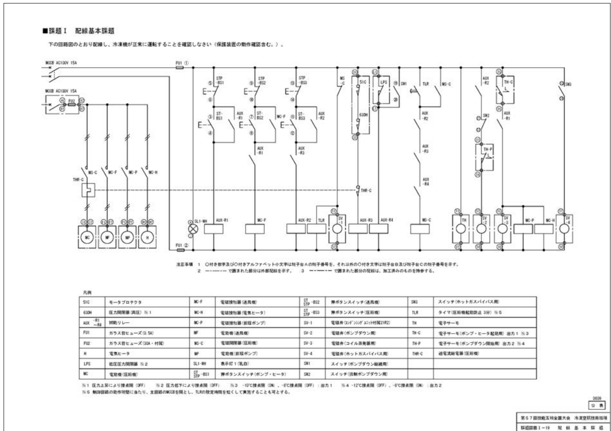
公表課題 配線基本課題
