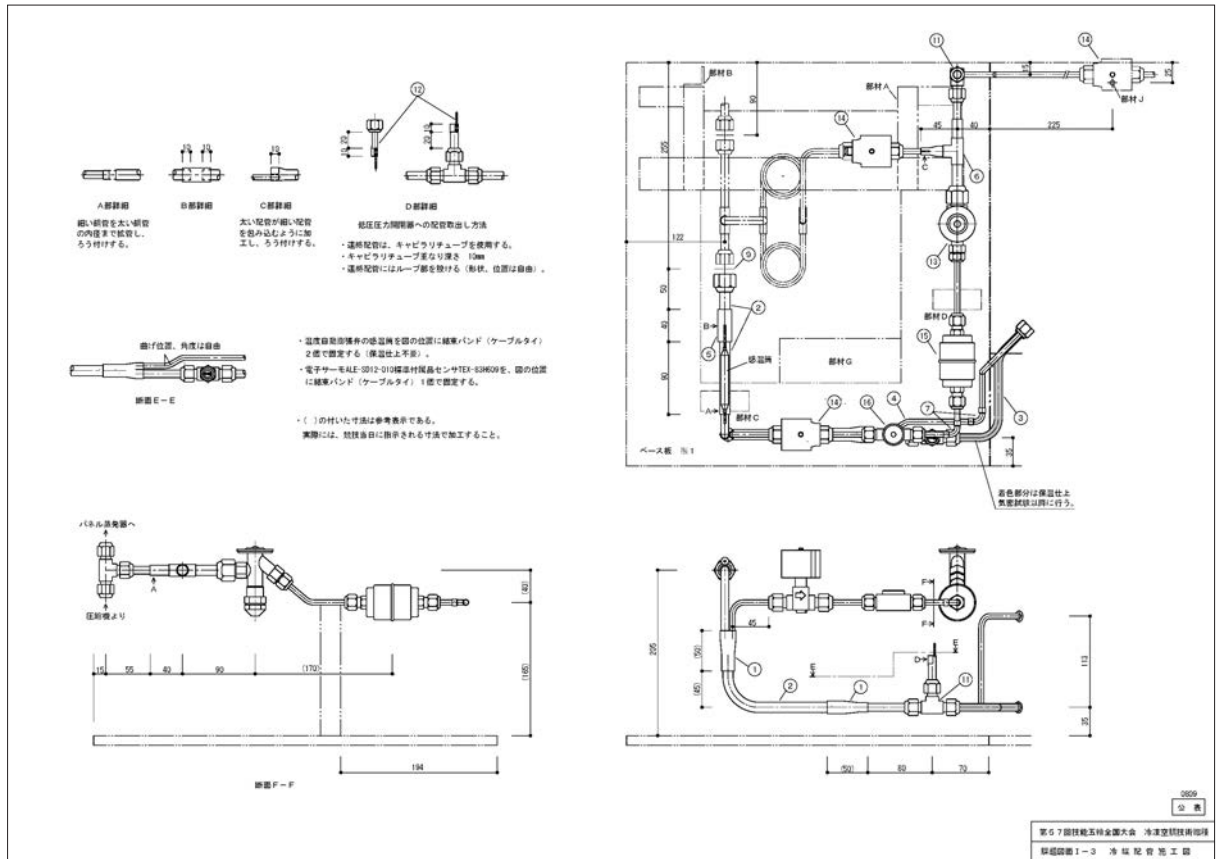
公表課題 冷媒配管施工図
