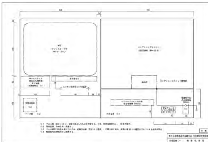
機器配置図
