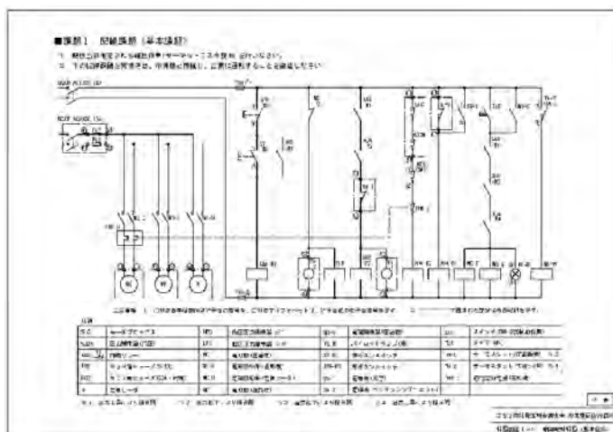
制御配線課題（基本回路）
